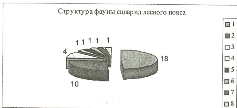
Рис.2. Структура фауны сциарид лесного пояса
