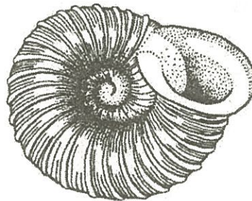
Рисунок 1. Раковина Vallonia ( Vallonia ) costata (Muller, 1774)
