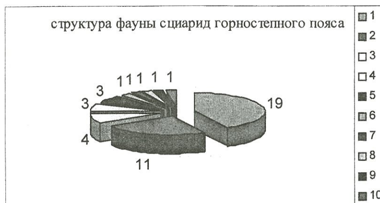
Рис.1. Структура фауны сциарид горностепного пояса.
