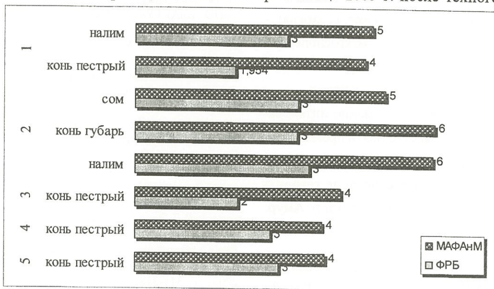
Рис. 3. Обсемененность жабер рыб МАФАНМ и ФРБ, выловленных в период ледостава 2006 г.:
