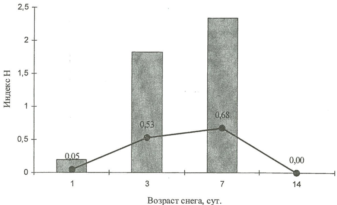
Рис. 2. Динамика разнообразия биогеоценотической структуры ИП косули в градиенте снежного покрова в степных лесах
