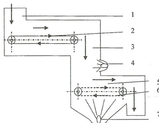
Рисунок-1. Установка для увлажнения хлопкового волокна
