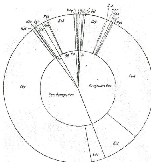
Рис.1. Диаграмма состава инфраотряда бибиоморф современной фауны; показаны надсемейства и семейства в виде секторов круга, размеры которых соответствуют количеству видов данного таксона (1 дуга равен 21 виду); в центре круга показаны надсемейства, по окружности семейства (по Родендорфу).
