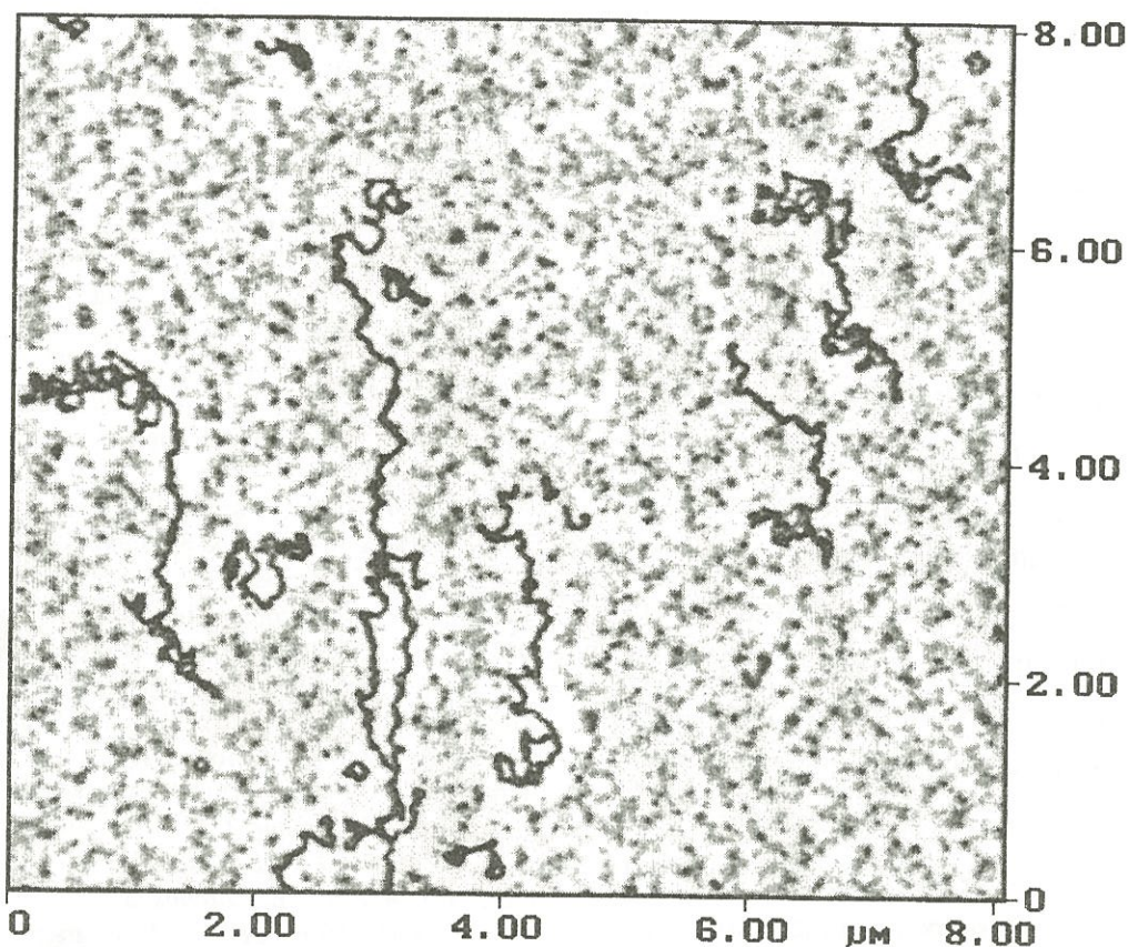
Рис. 3. Молекулы ДНК бактериофага Т4 адсорбированы из буфера в присутствии бромид ацетилтриметиламмония на слюду.
