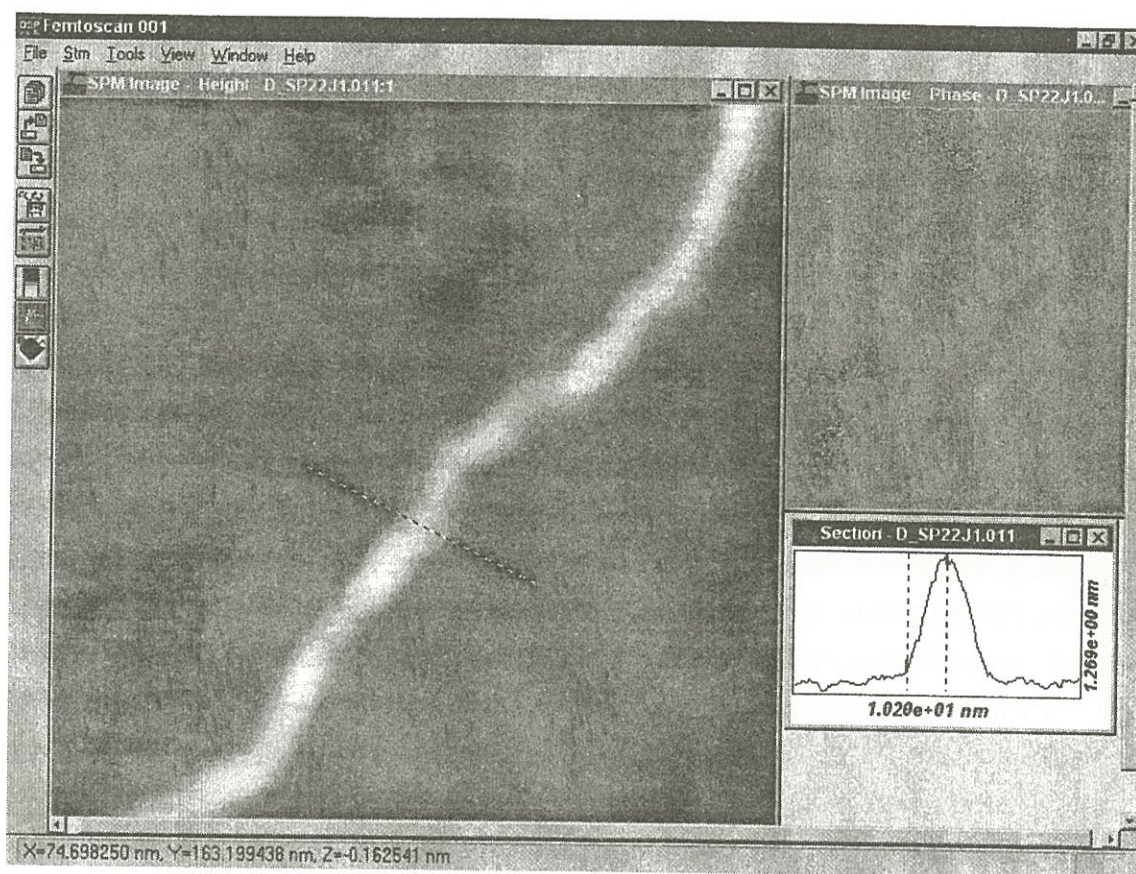
Рис. 2. Фрагмент молекулы ДНК, адсорбированной на слюду. АСМ-исследование, режим прерывистого контакта Размер основного кадра 0,2 \times 0,2 \text{ мкм}^2
