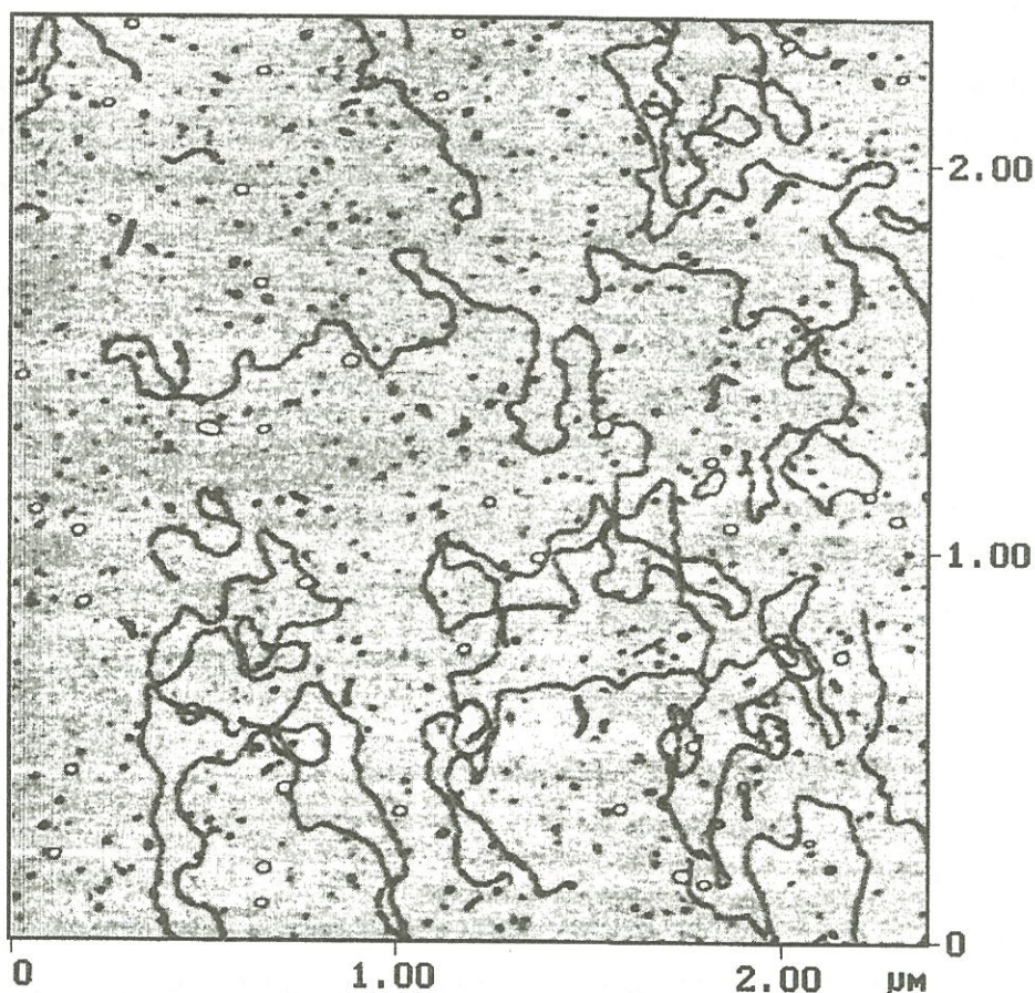
Рис. 1. Молекулы ДНК контрастированы уранилацетатом и адсорбированы на слюду. АСМ-исследование, контактный режим. Размер кадра 2,3* 2,3 мкм 2
