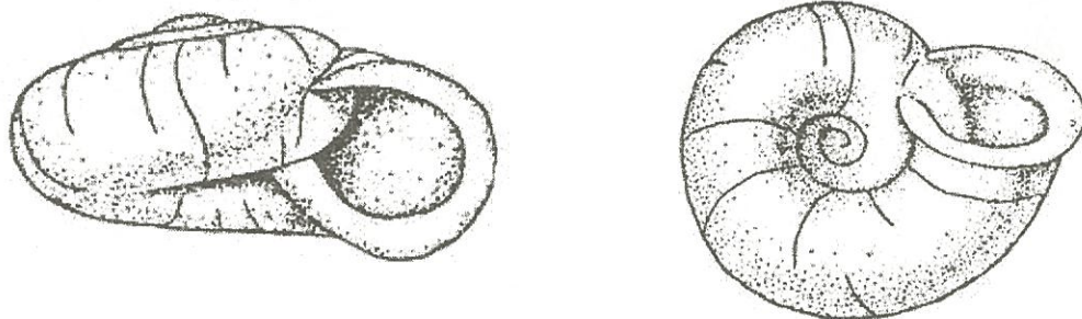
Рисунок 3. Раковина Vallonia (Vallonia) pulchella (Muller, 1774)
